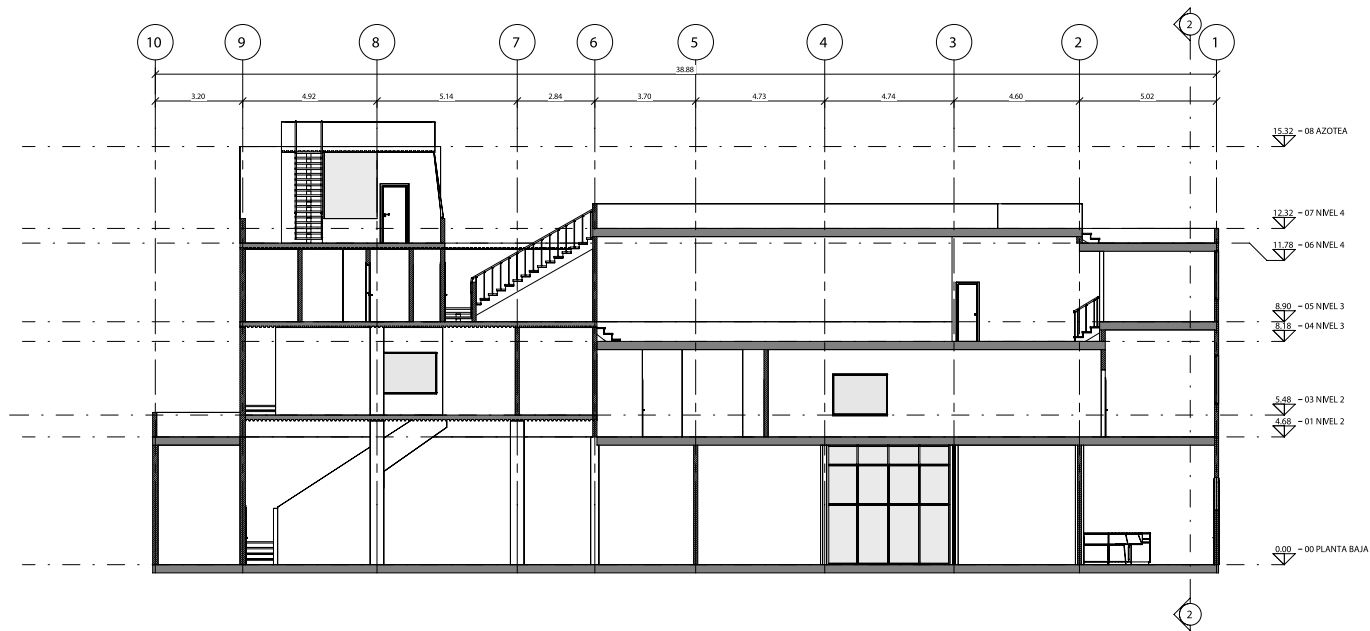
1 Sección 1 A10-02 1:100
