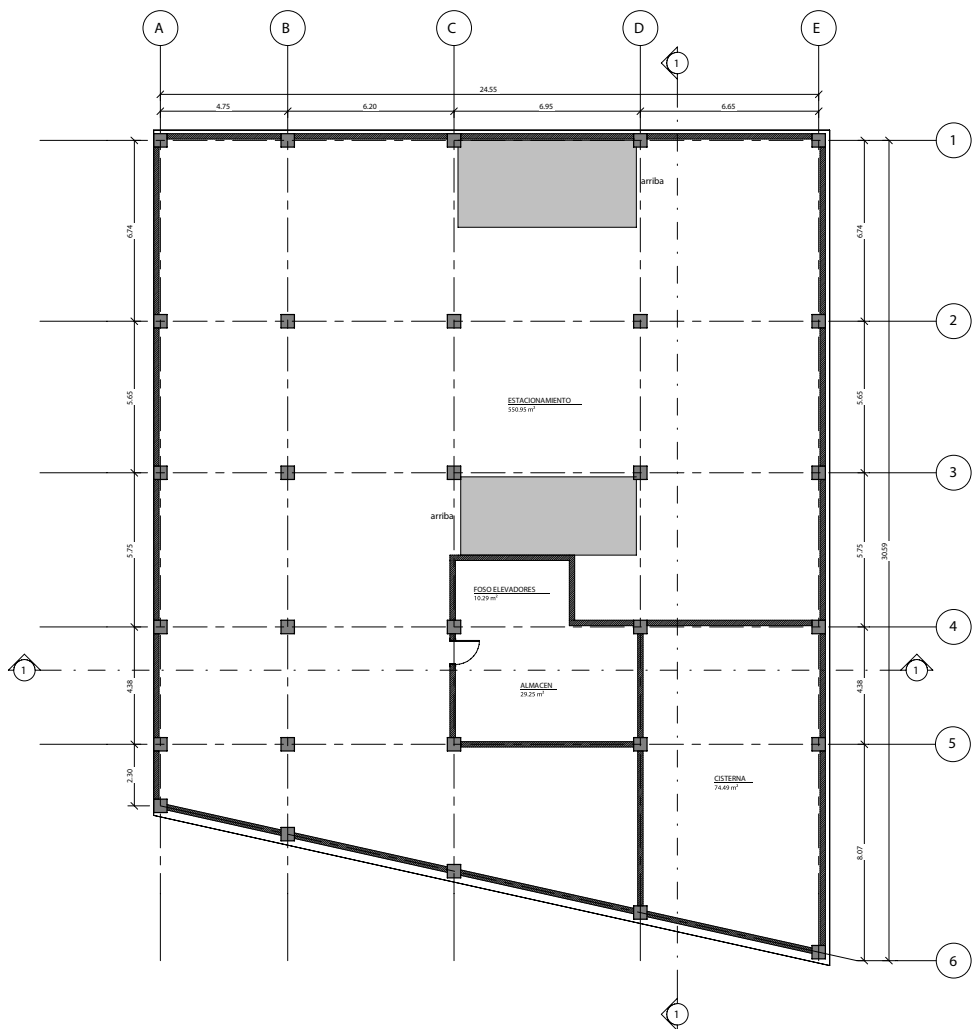
01 SOTANO 3 ARG.01 1:100
