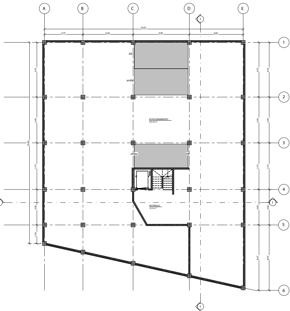
02 SOTANO 2 ARG.02 1:100
