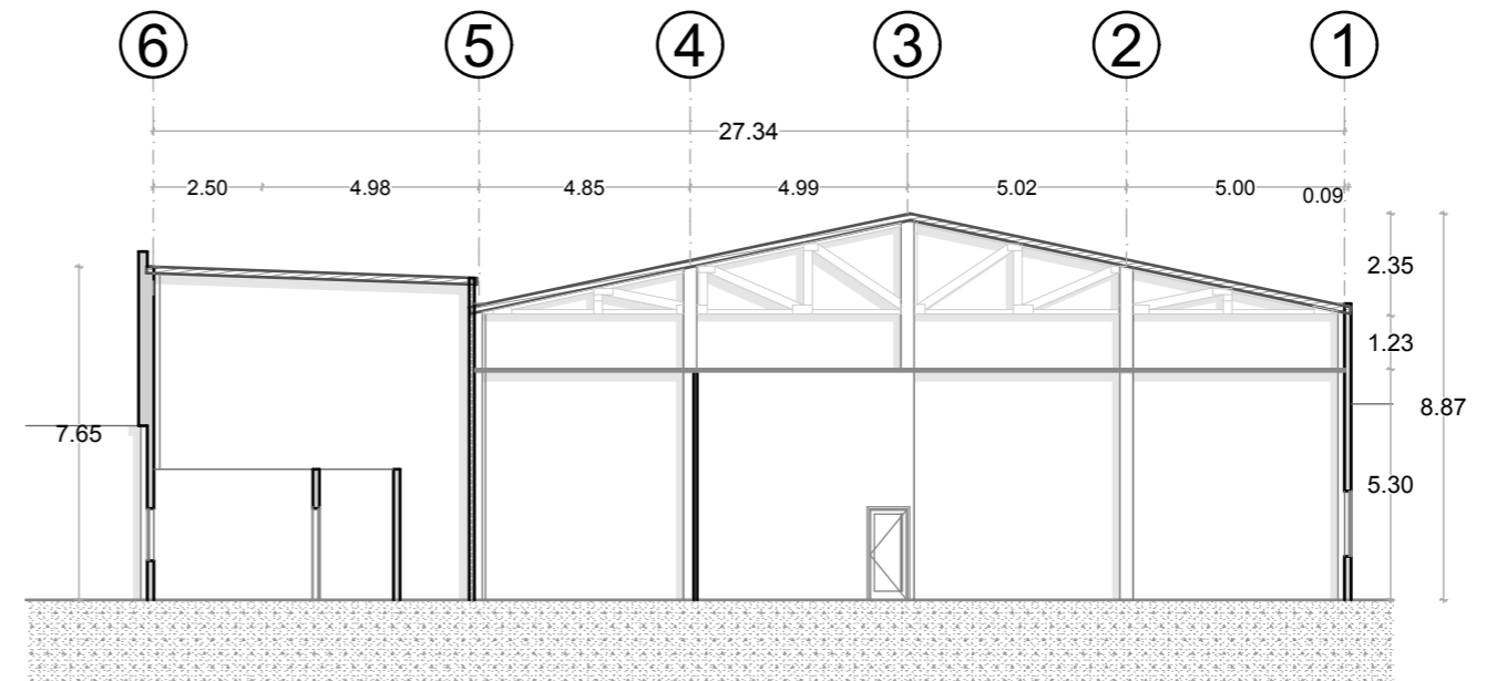
CORTE
