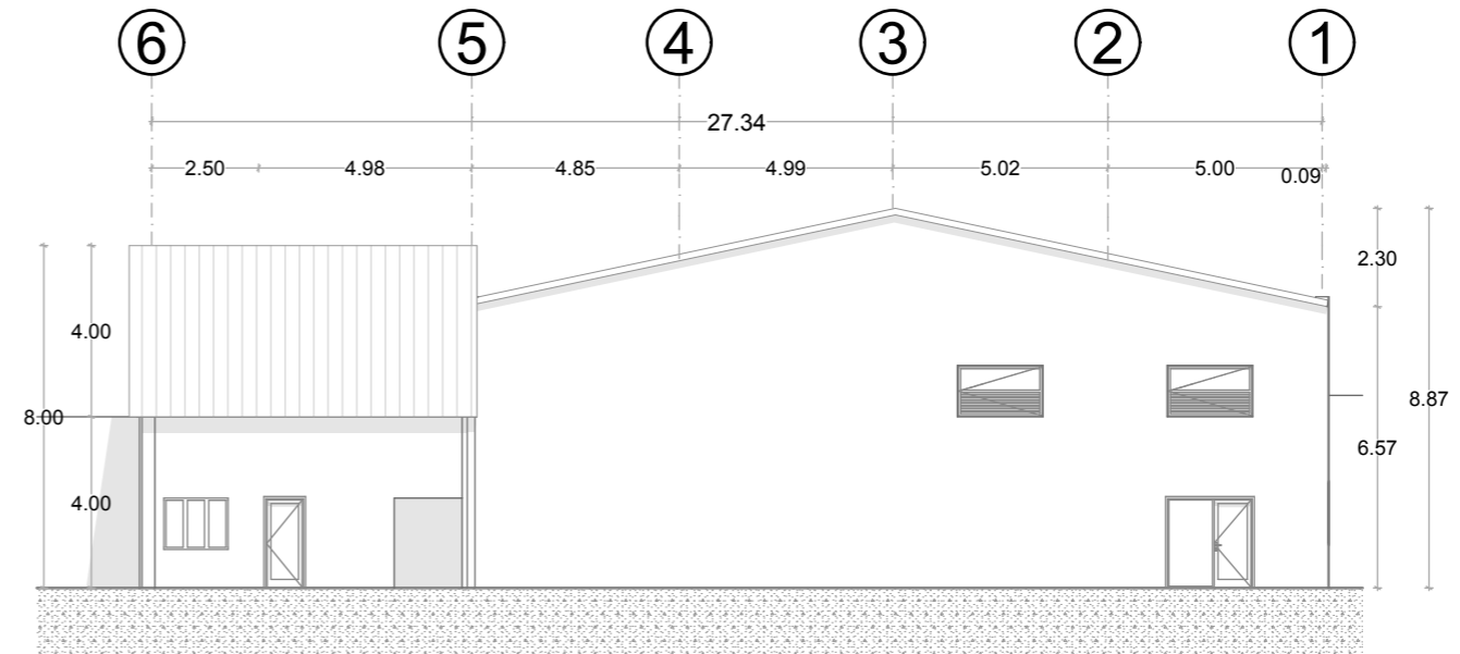
FACHADA
