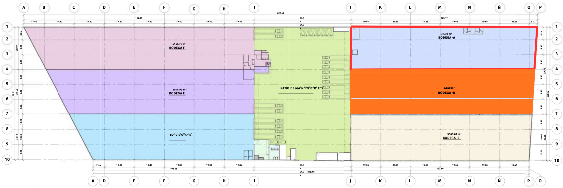
1 PLANTA BAJA ARQ-011:500
